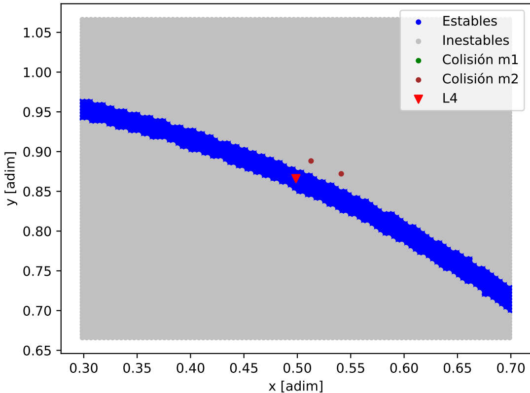
Mapa de estabilidad - WASP-47_WASP-47_c
