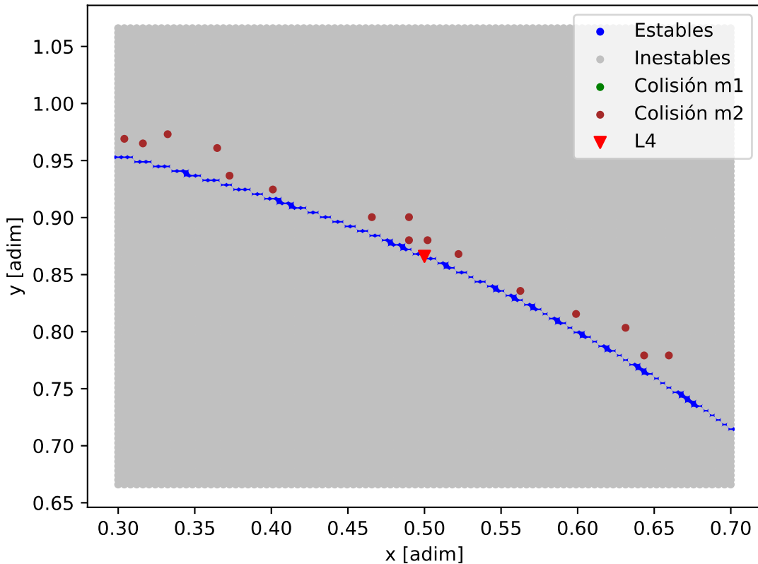
Mapa de estabilidad - WASP-47_WASP-47_e
