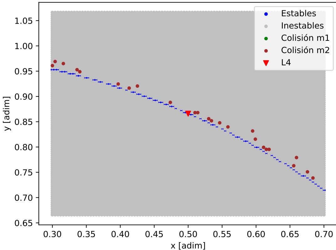
Mapa de estabilidad - \rho_{CrB\_rho\_CrB\_e}
