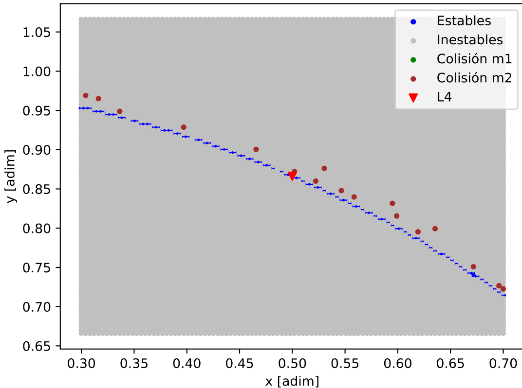
Mapa de estabilidad - \tau_{Cet} \tau_{Cet_f}
