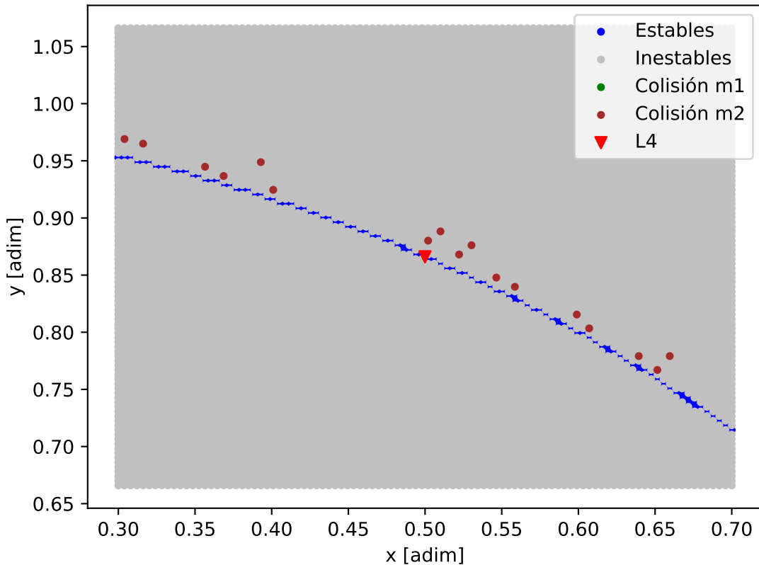
Mapa de estabilidad - GJ_9827_GJ_9827_b
