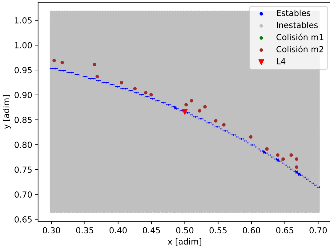
Mapa de estabilidad - HD_110067_HD_110067_f
