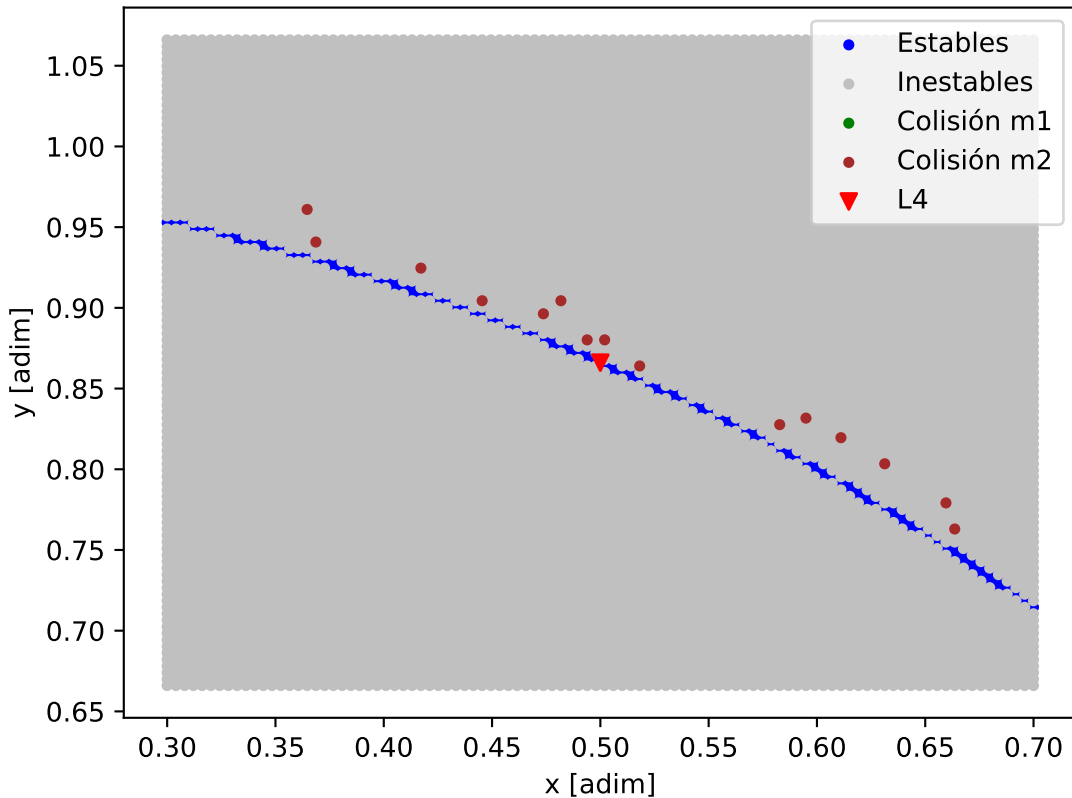
Mapa de estabilidad - HD_110067_HD_110067_g
