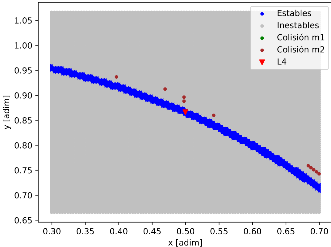
Mapa de estabilidad - HD_141399_HD_141399_b
