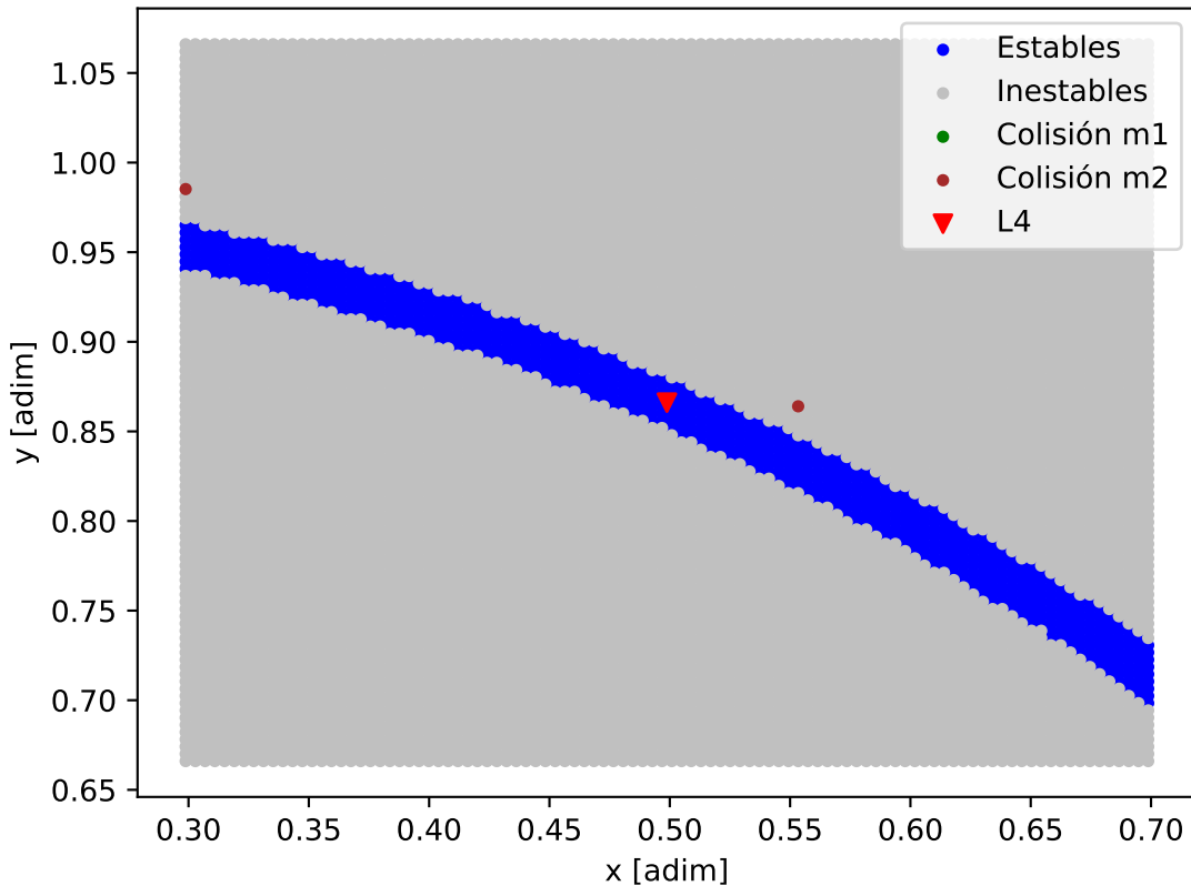
Mapa de estabilidad - HD_141399_HD_141399_c
