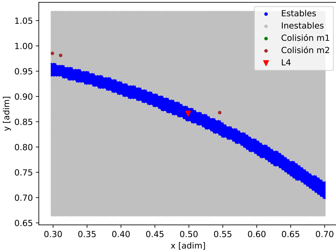
Mapa de estabilidad - HD_141399_HD_141399_d
