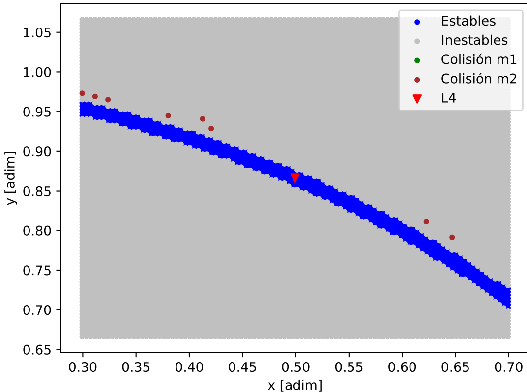
Mapa de estabilidad - HD_141399_HD_141399_e
