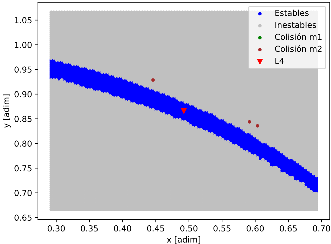
Mapa de estabilidad - HD_181433_HD_181433_c
