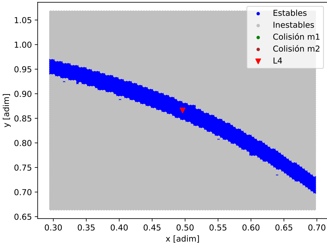
Mapa de estabilidad - HD_215152_HD_215152_e
