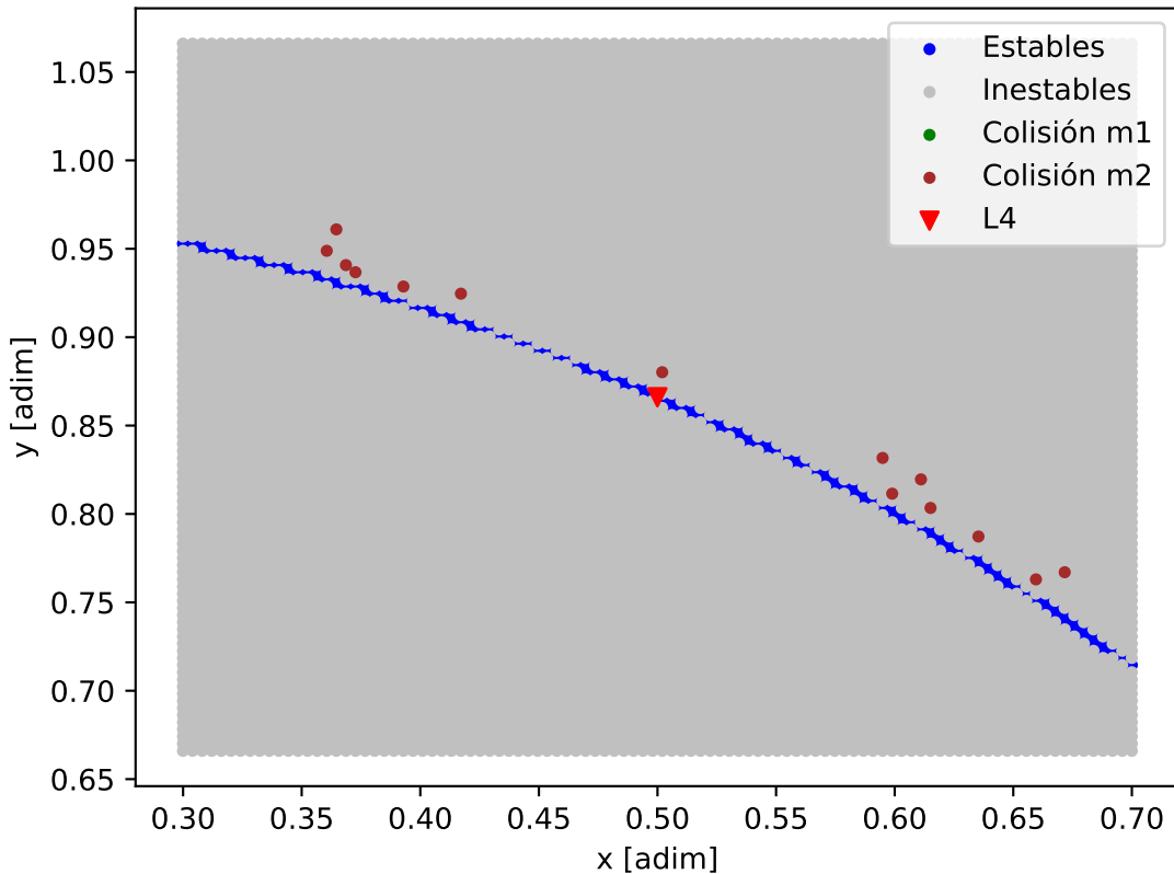
Mapa de estabilidad - HD_23472_HD_23472_b
