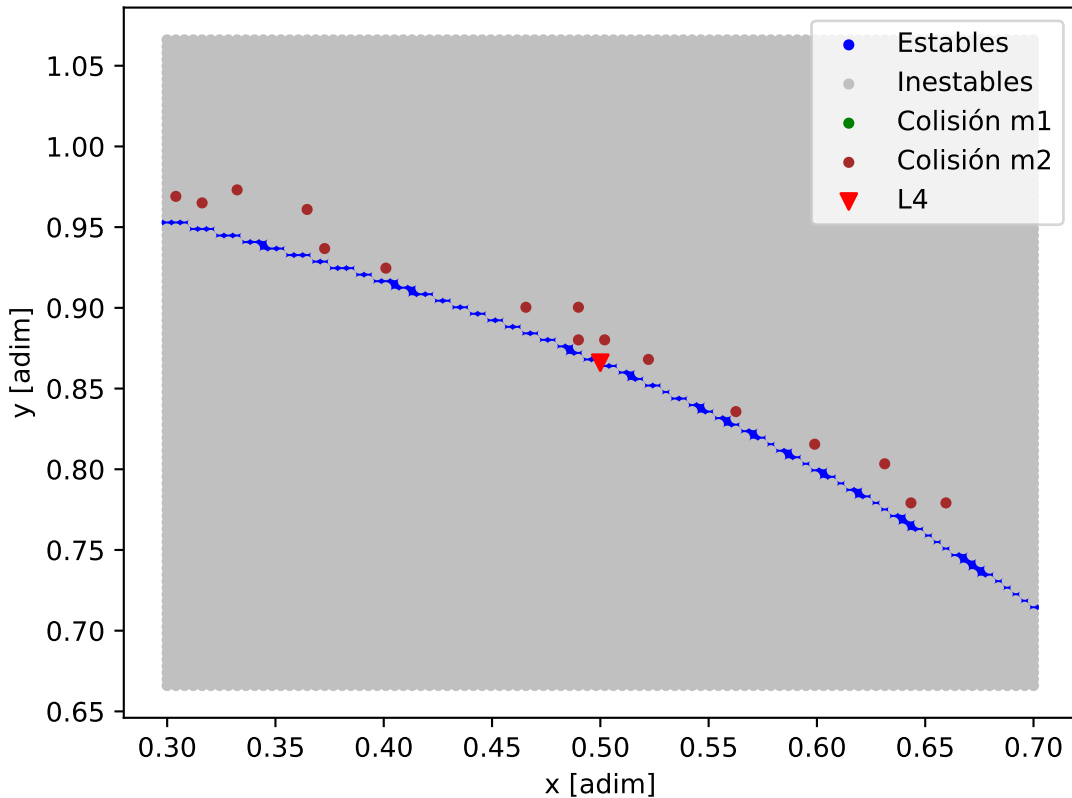
Mapa de estabilidad - HD_3167_HD_3167_d
