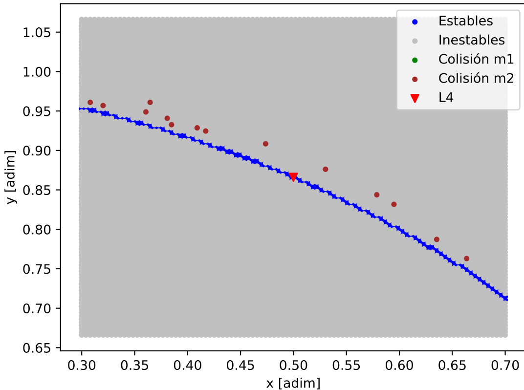
Mapa de estabilidad - HD_3167_HD_3167_e
