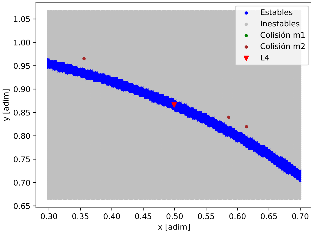
Mapa de estabilidad - HD_33142_HD_33142_b
