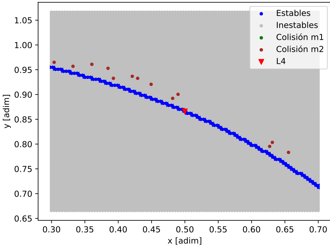
Mapa de estabilidad - HD_33142_HD_33142_d
