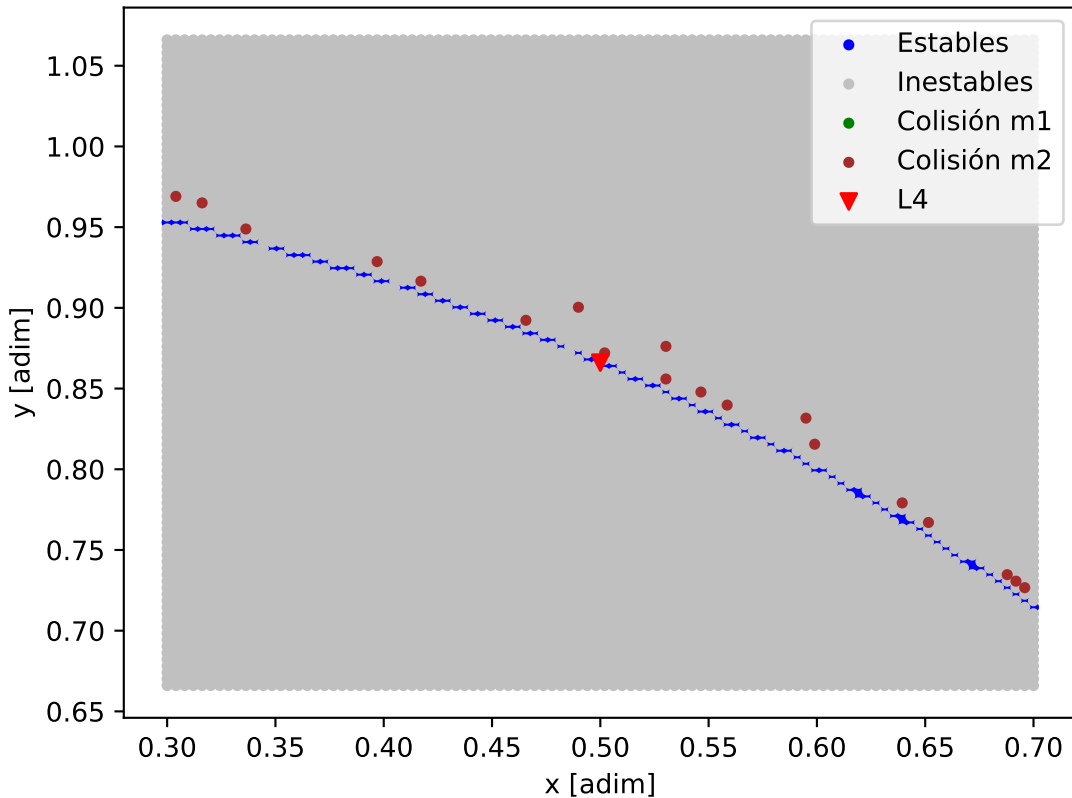
Mapa de estabilidad - HD_39194_HD_39194_b
