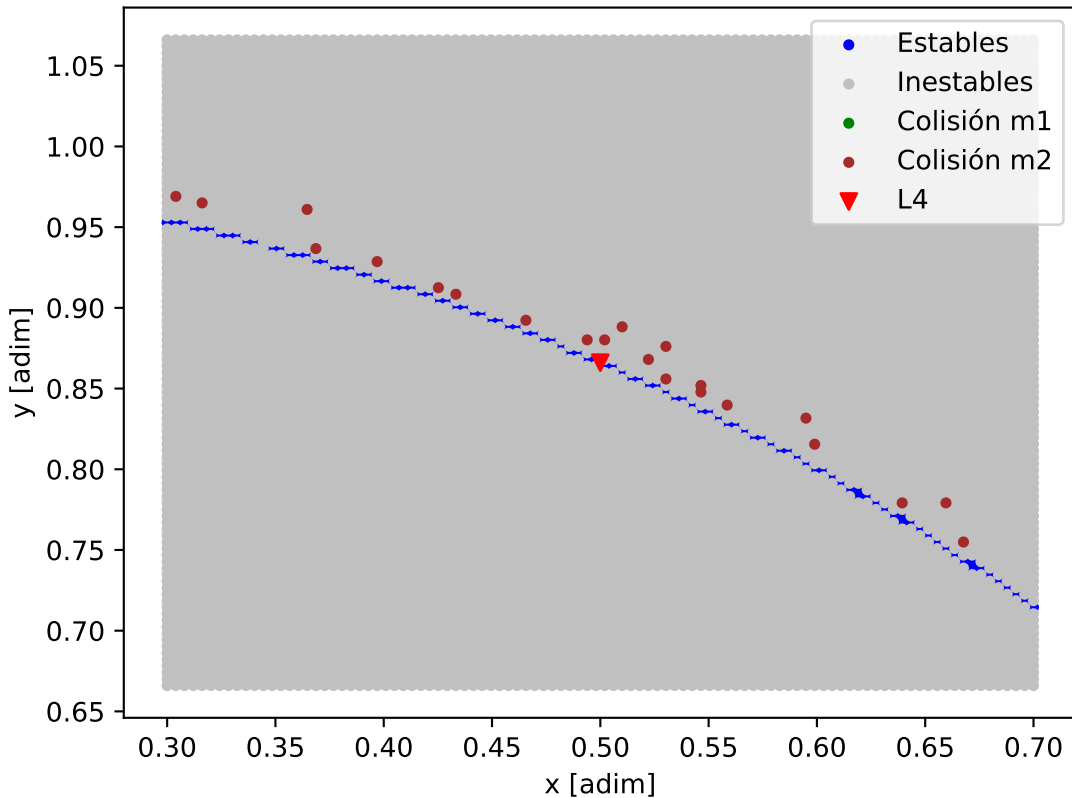
Mapa de estabilidad - HD_39194_HD_39194_d
