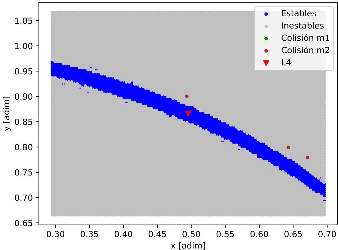
Mapa de estabilidad - HD_40307_HD_40307_b
