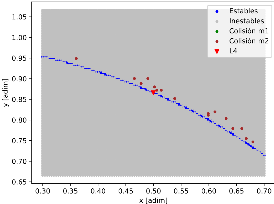
Mapa de estabilidad - HD_40307_HD_40307_g
