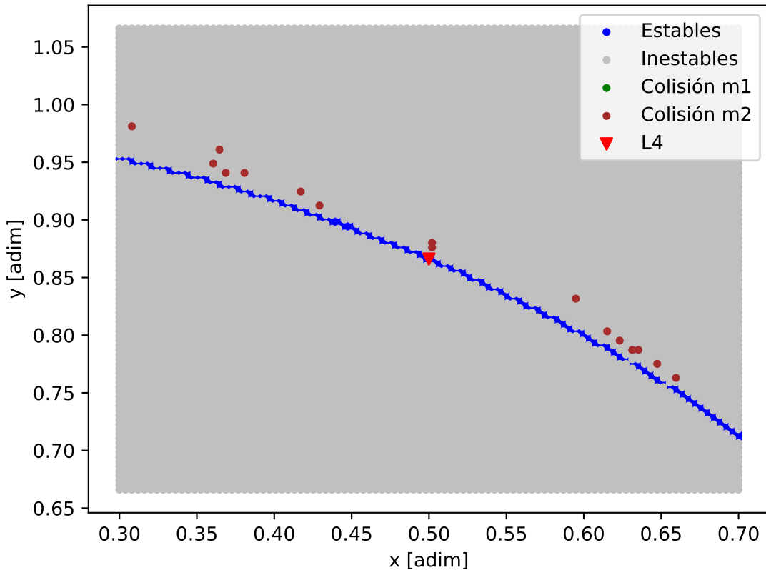
Mapa de estabilidad - HD_48948_HD_48948_d
