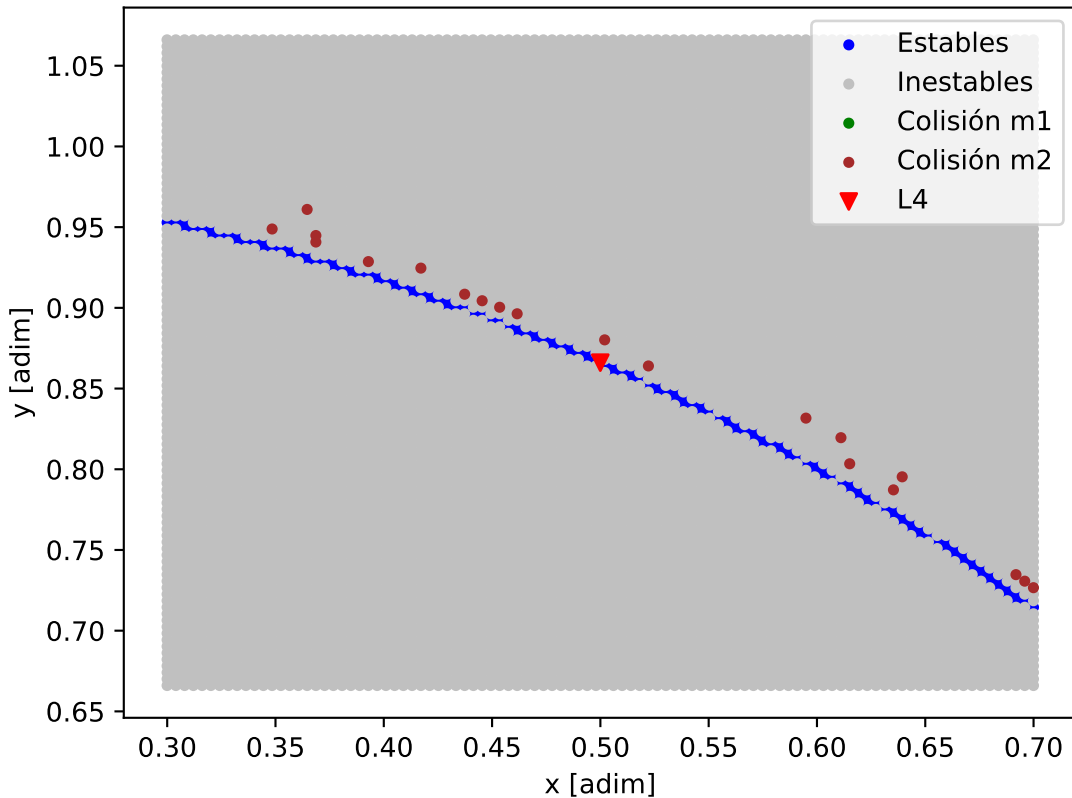
Mapa de estabilidad - HD_69830_HD_69830_c
