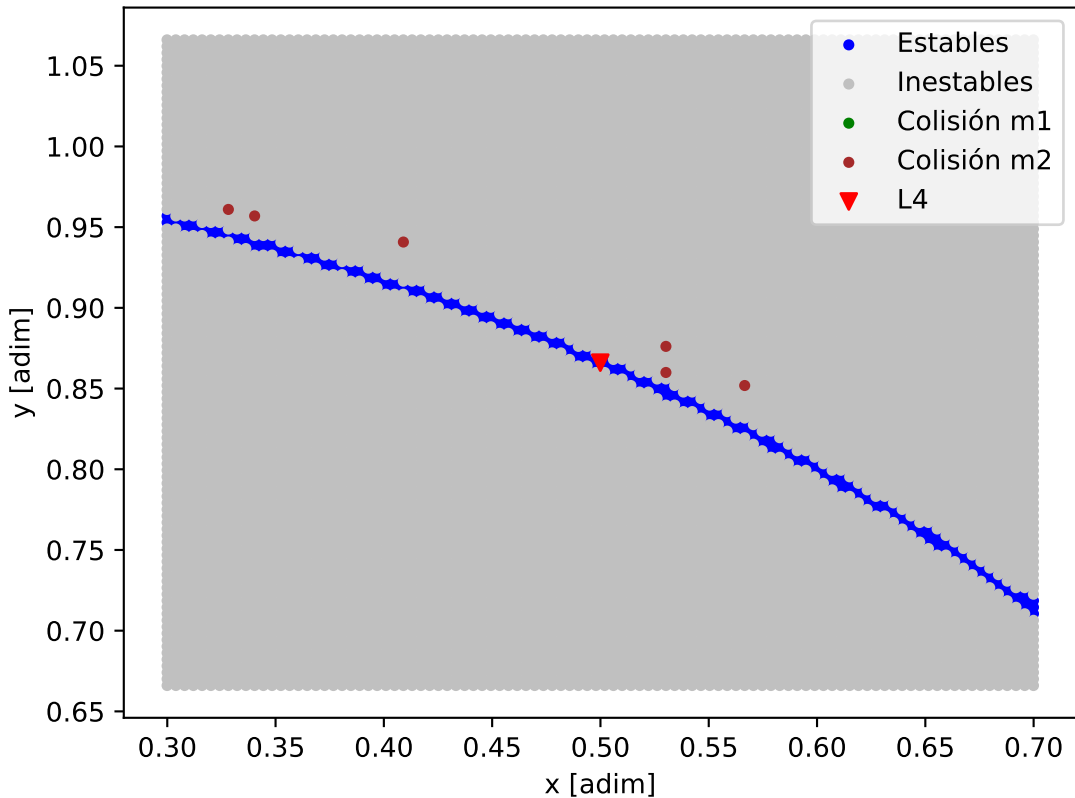
Mapa de estabilidad - K2-136_K2-136_c
