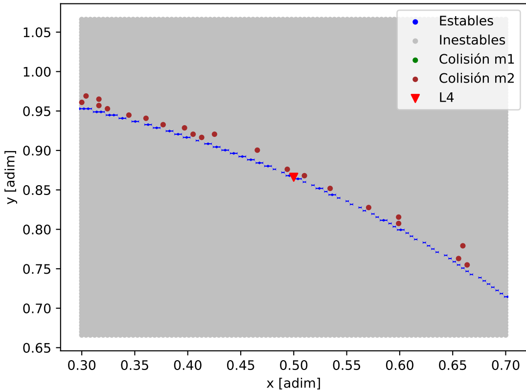
Mapa de estabilidad - K2-233_K2-233_b
