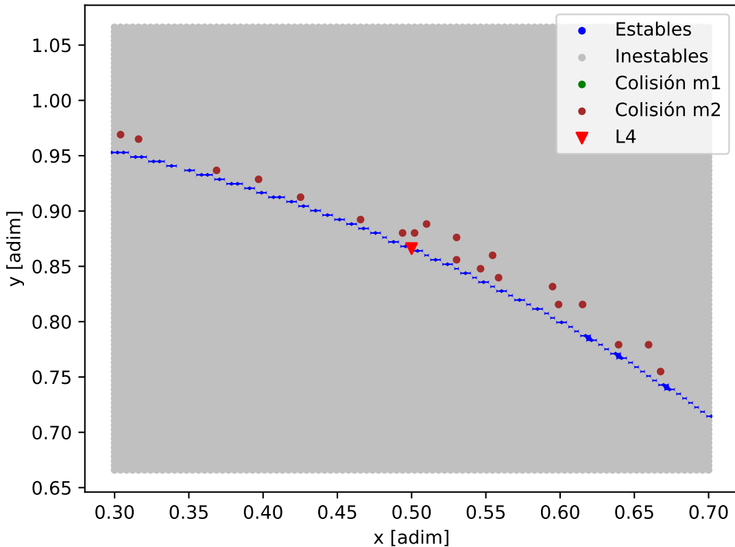
Mapa de estabilidad - K2-233_K2-233_c
