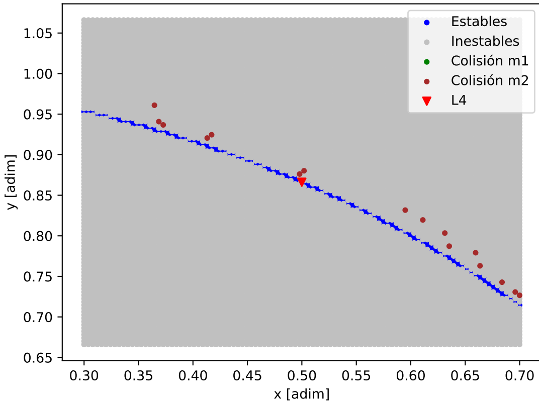
Mapa de estabilidad - K2-285_K2-285_b
