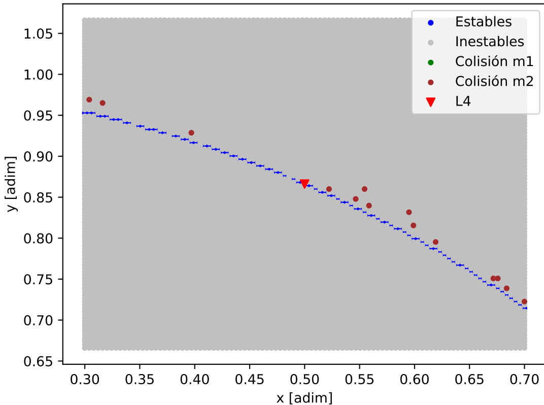
Mapa de estabilidad - Kepler-167_Kepler-167_b
