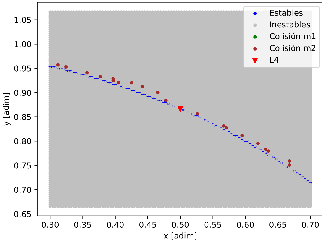
Mapa de estabilidad - Kepler-167_Kepler-167_d
