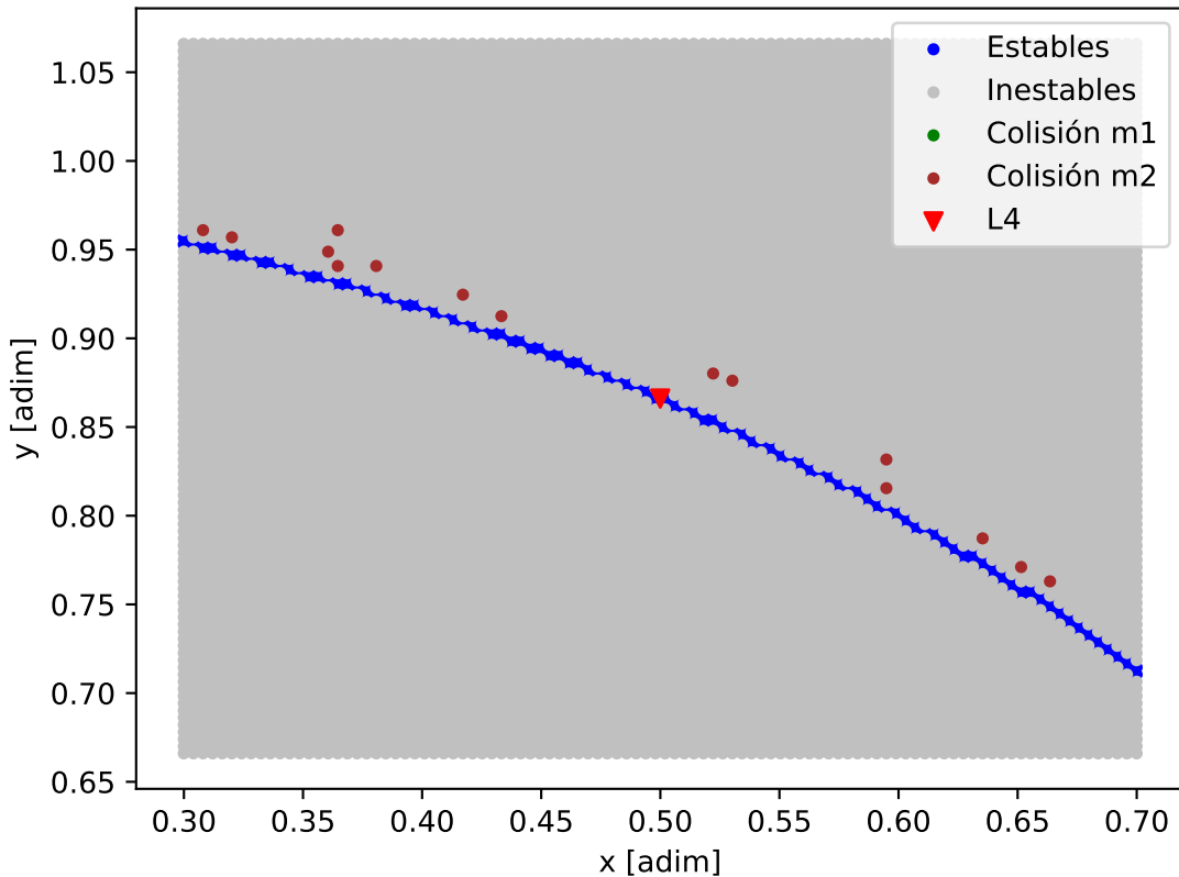
Mapa de estabilidad - Kepler-247_Kepler-247_c
