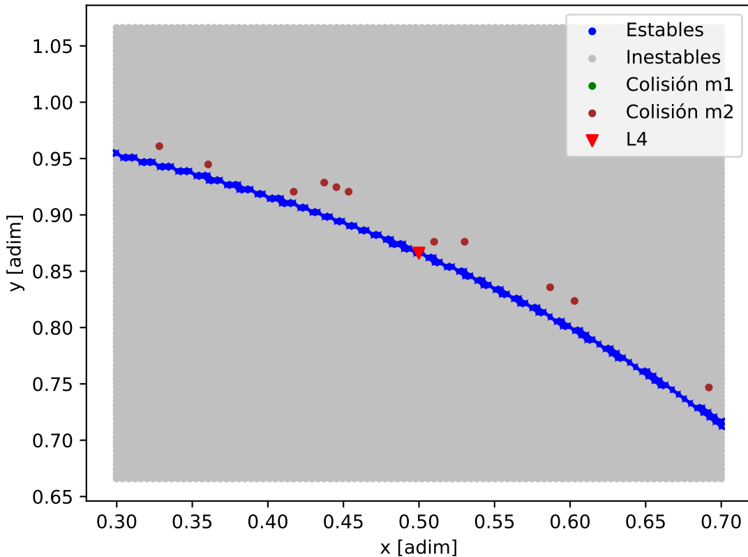
Mapa de estabilidad - Kepler-411_Kepler-411_b
