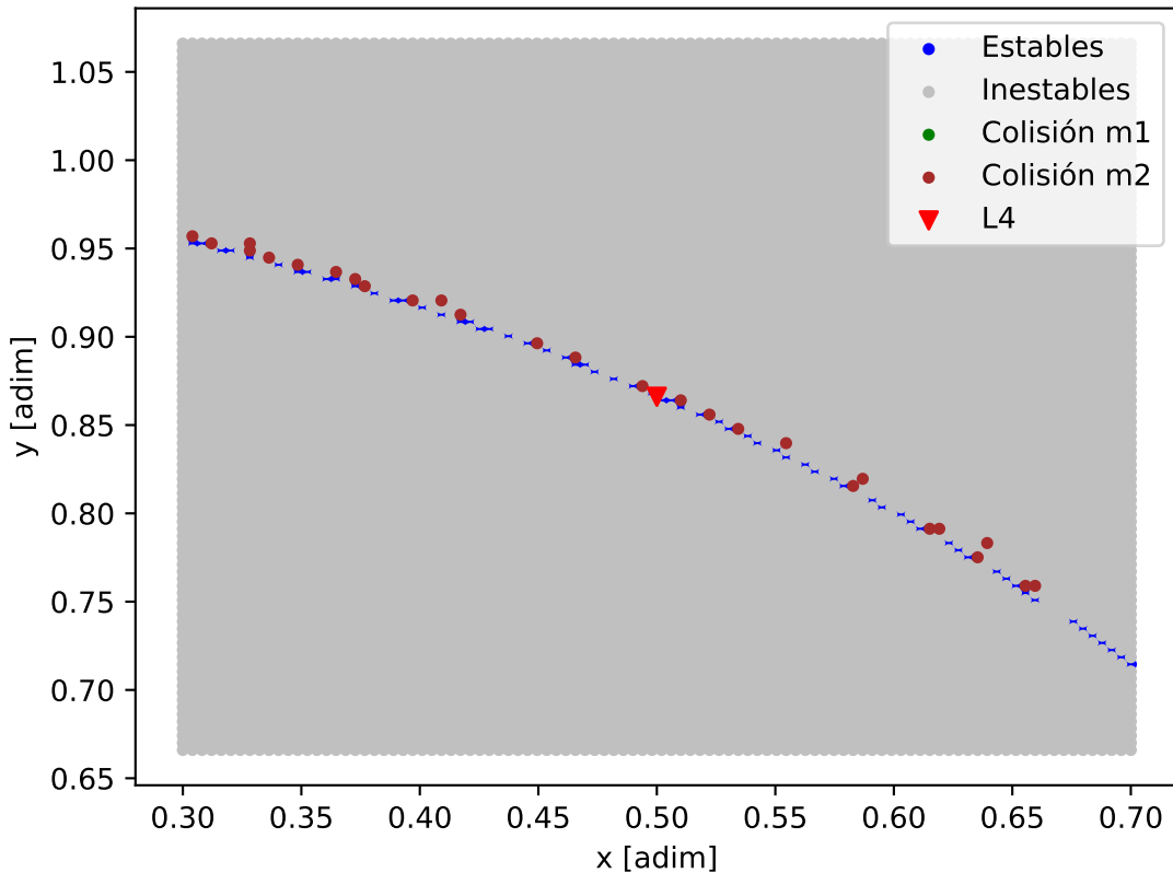
Mapa de estabilidad - Kepler-444_Kepler-444_d
