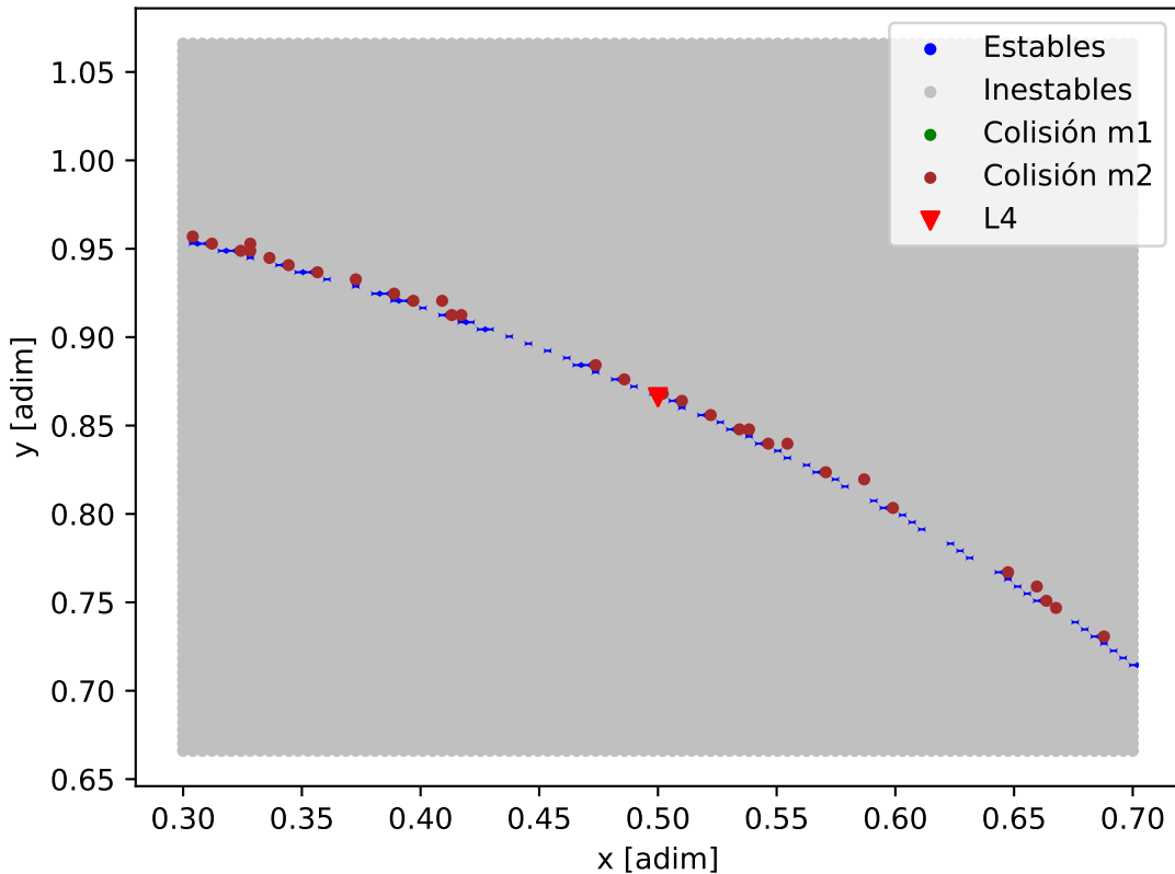
Mapa de estabilidad - Kepler-444_Kepler-444_e
