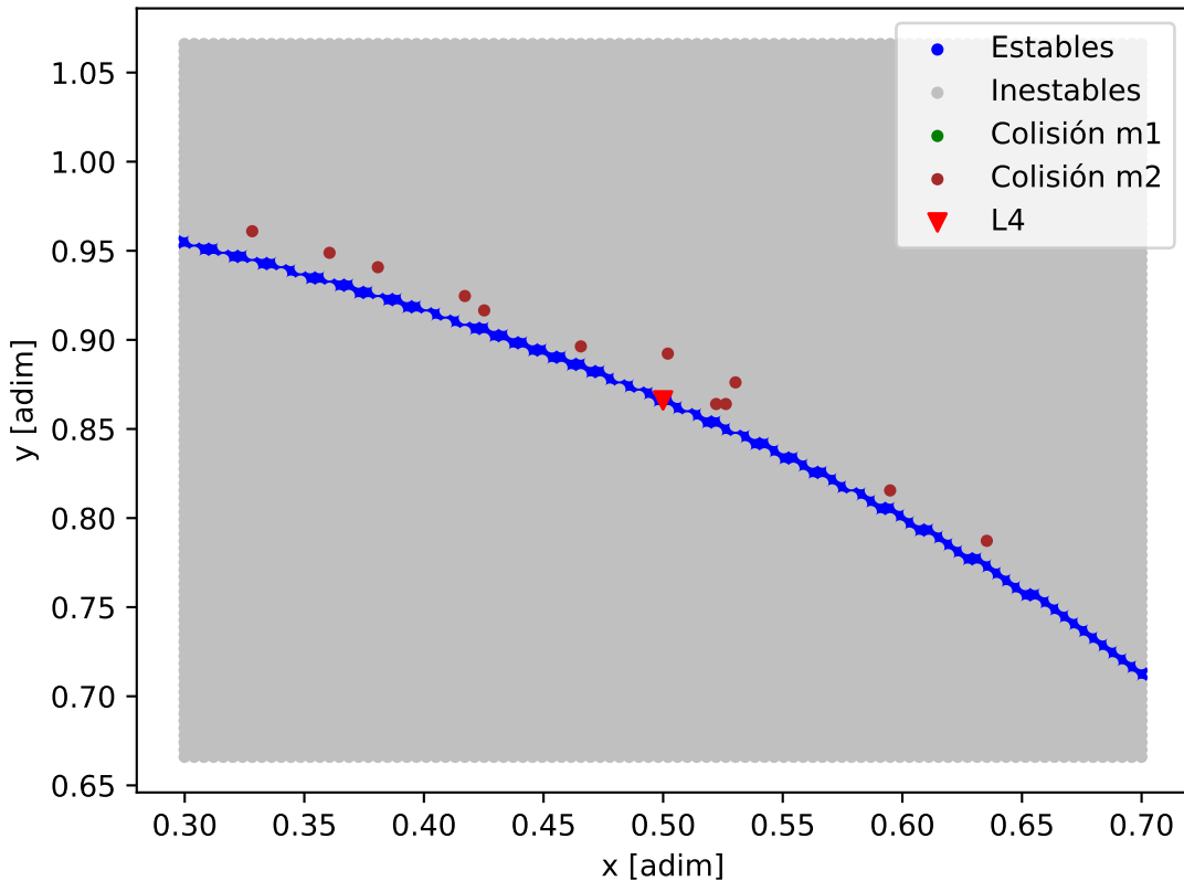
Mapa de estabilidad - Kepler-62_Kepler-62_d
