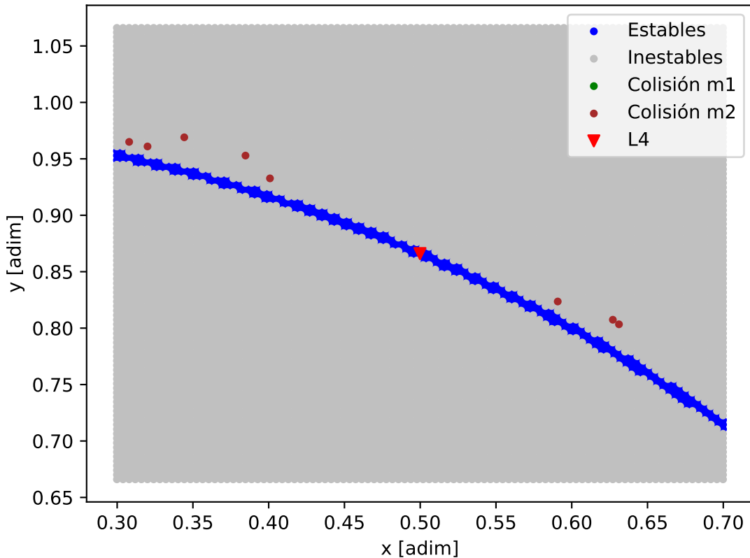
Mapa de estabilidad - Kepler-62_Kepler-62_e
