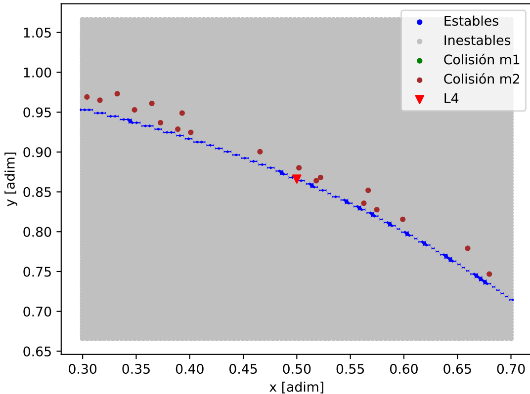
Mapa de estabilidad - Kepler-80_Kepler-80_c
