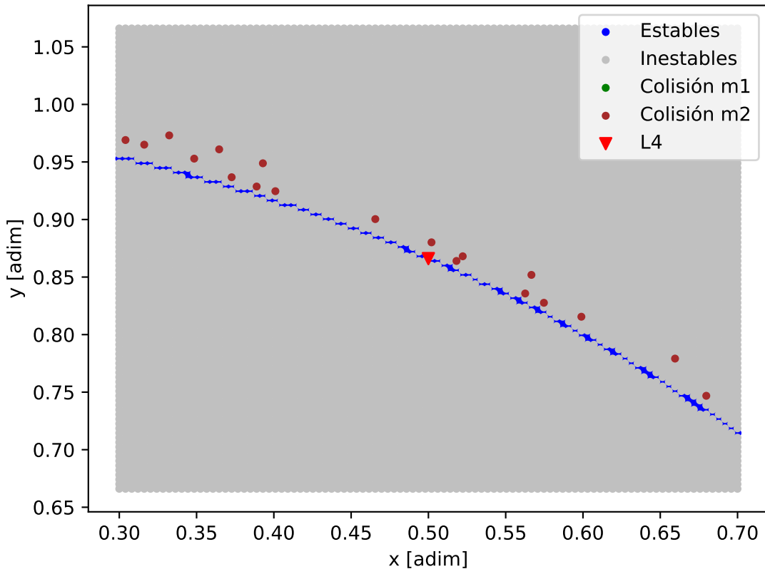
Mapa de estabilidad - Kepler-80_Kepler-80_d
