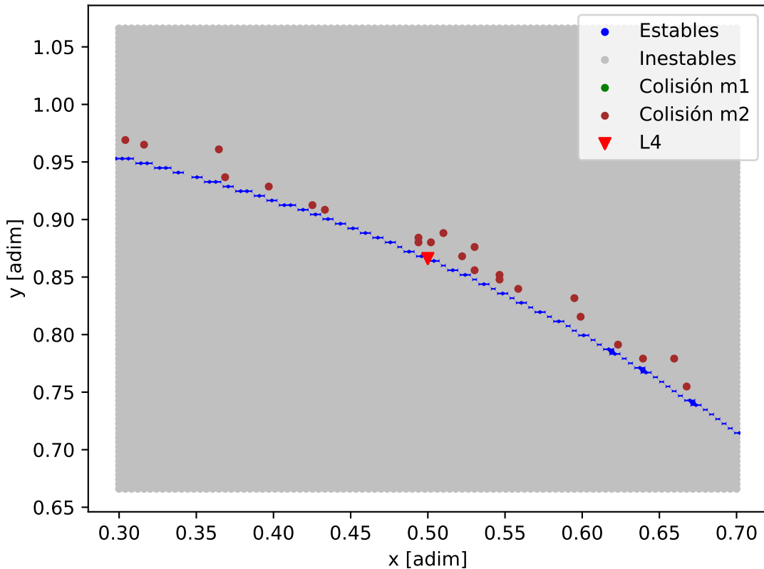
Mapa de estabilidad - TOI-1246_TOI-1246_d
