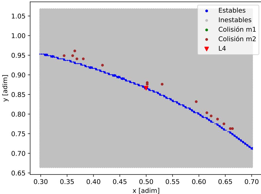
Mapa de estabilidad - TOI-125_TOI-125_d
