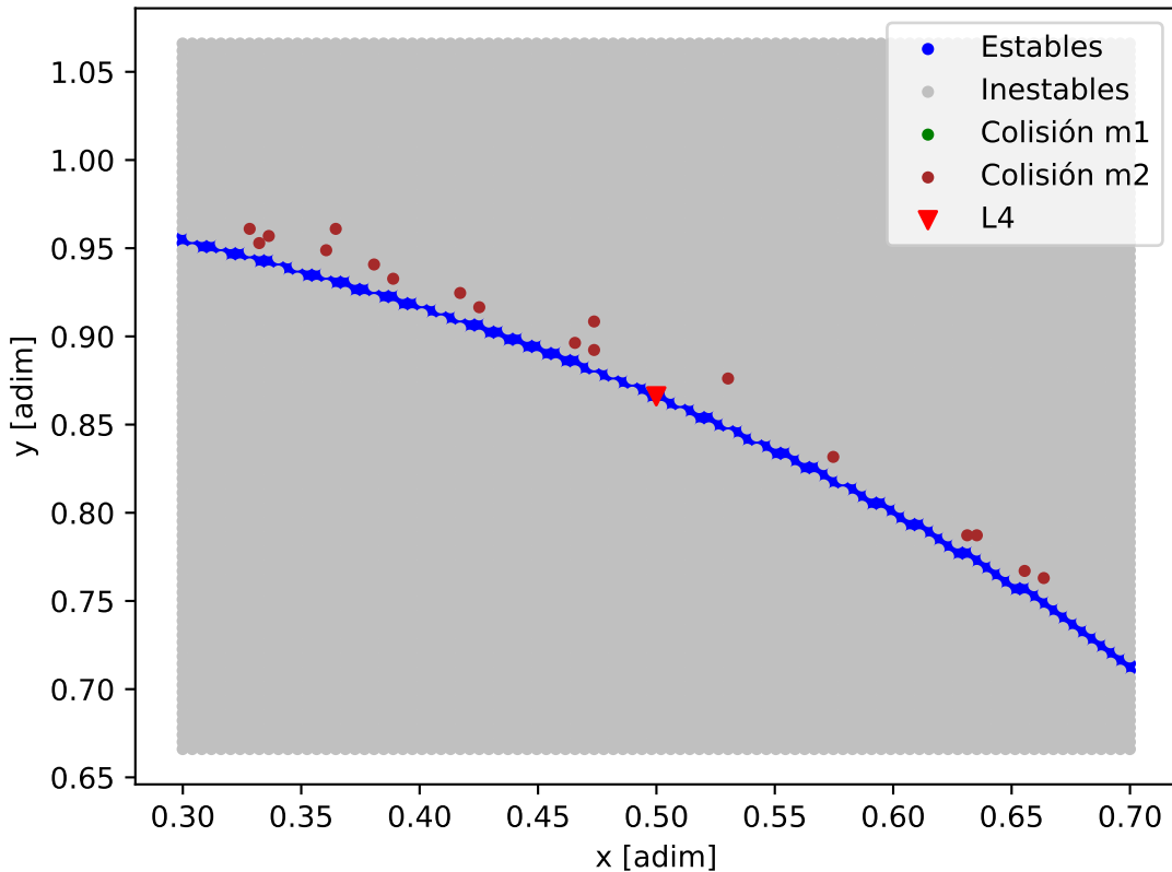
Mapa de estabilidad - TOI-1260_TOI-1260_c
