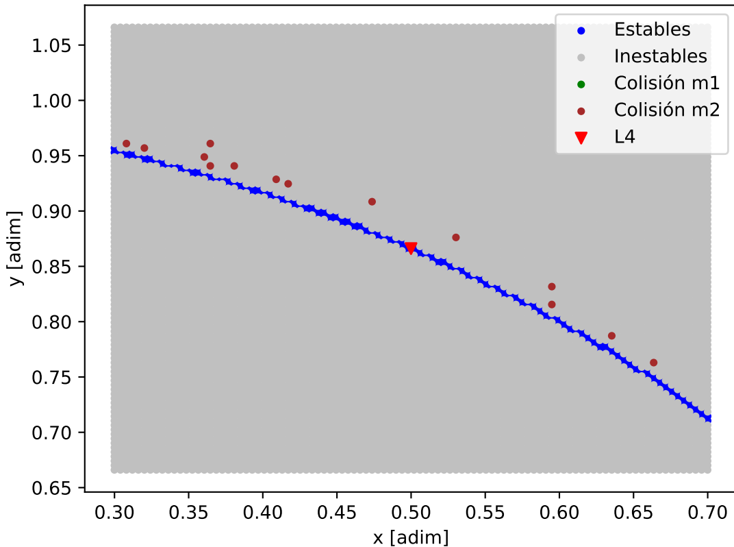
Mapa de estabilidad - TOI-1260_TOI-1260_d
