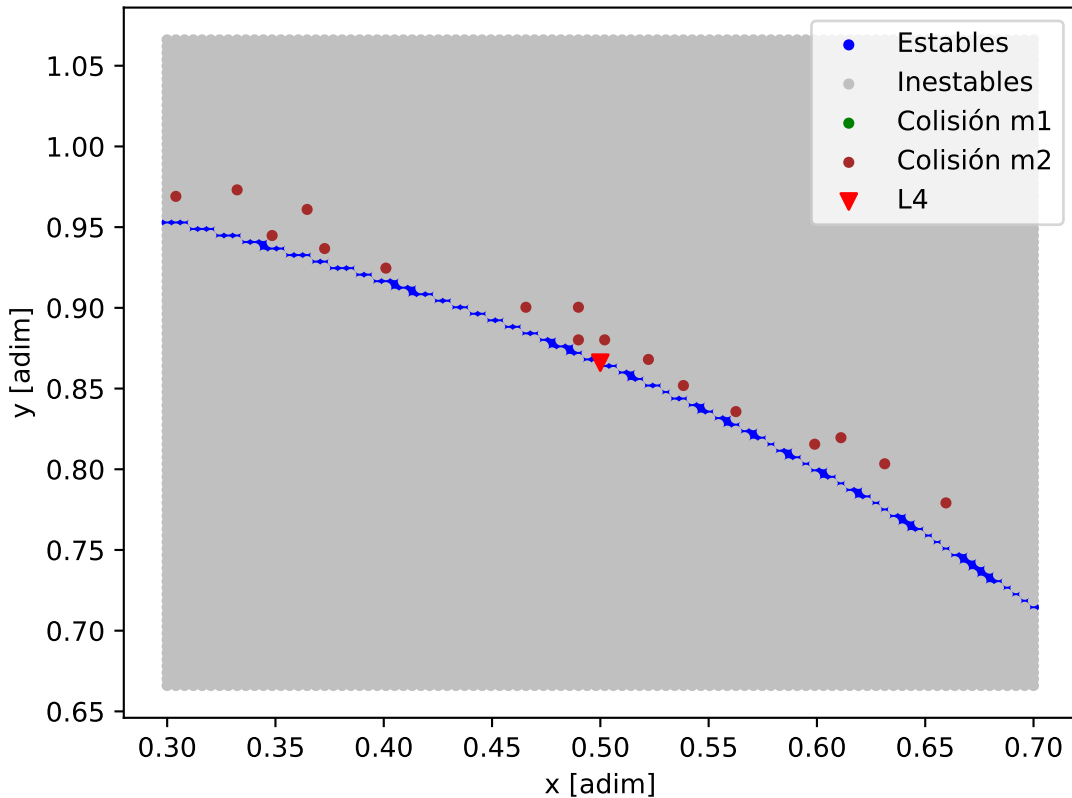
Mapa de estabilidad - TOI-178_TOI-178_f
