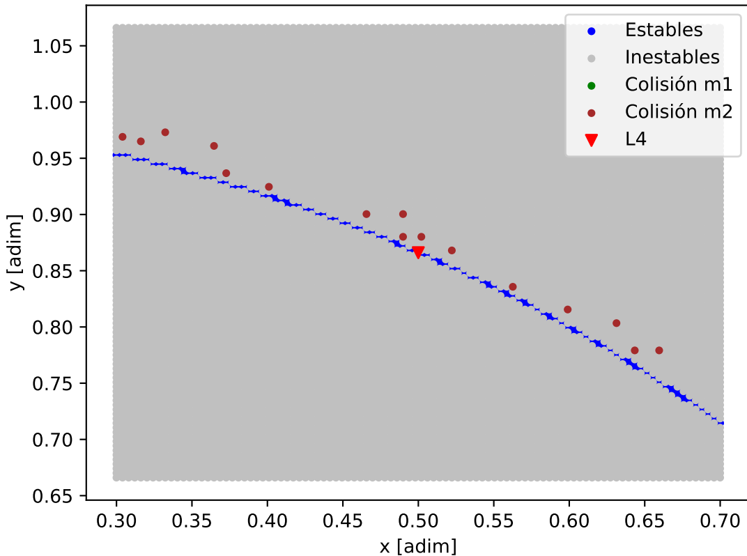
Mapa de estabilidad - TOI-2076_TOI-2076_c
