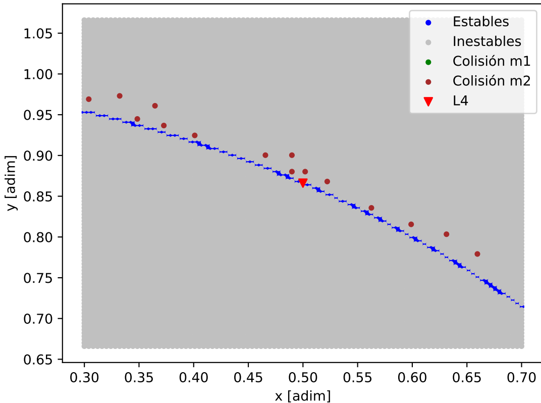
Mapa de estabilidad - TOI-2076_TOI-2076_d
