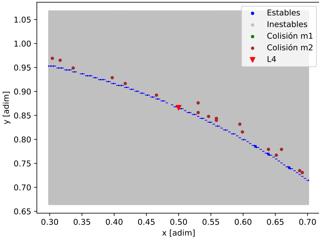
Mapa de estabilidad - TOI-2076_TOI-2076_e
