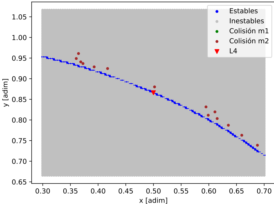
Mapa de estabilidad - TOI-4010_TOI-4010_b
