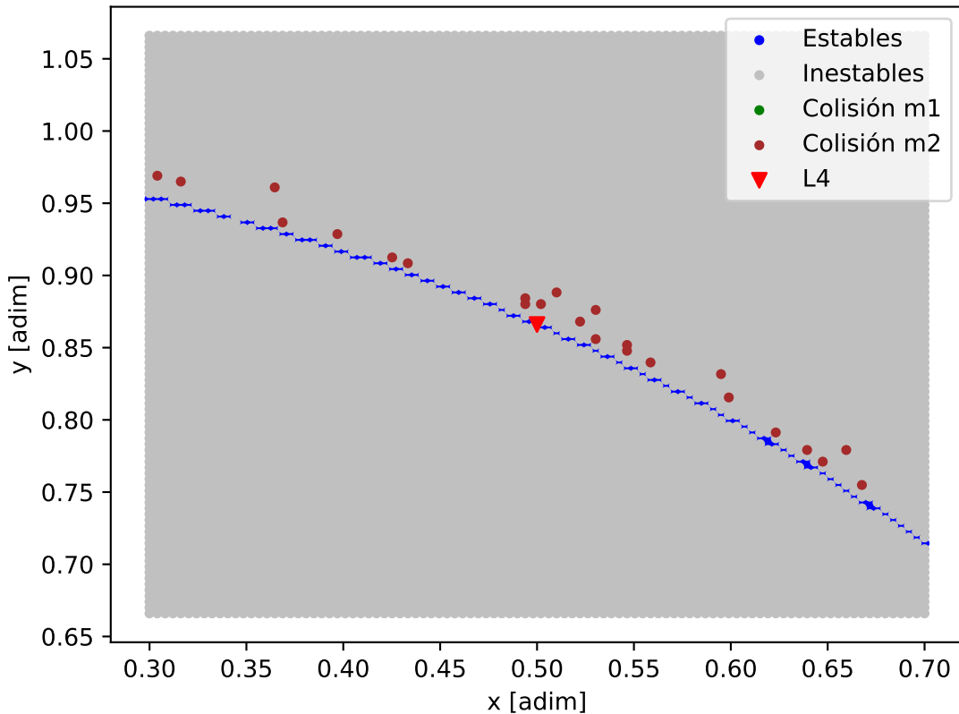
Mapa de estabilidad - TOI-5789_TOI-5789_c
