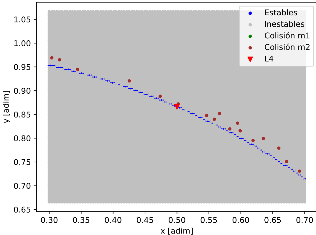
Mapa de estabilidad - V1298_Tau_V1298_Tau_c
