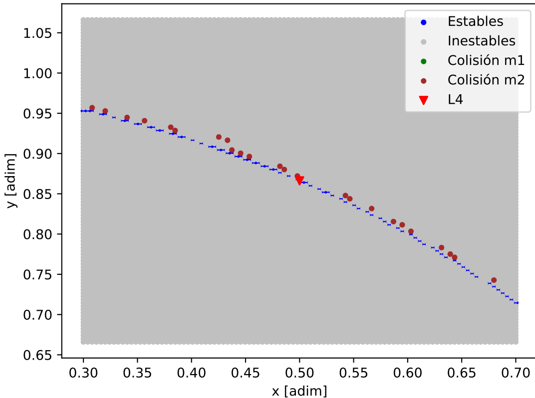
Mapa de estabilidad - Barnard's_star_Barnard_b
